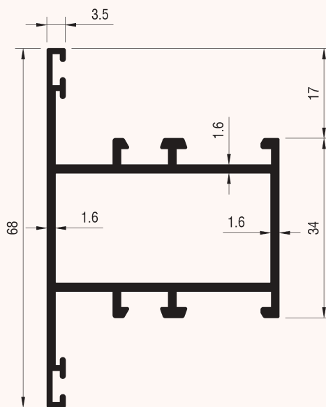
Profile Code : FD-6008 Unit Weight : 0.958 kg/m Perimeter : 337.9 mm
