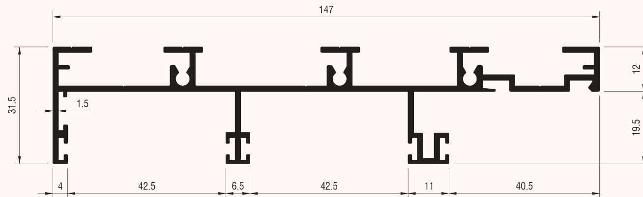
Profile Code : SD-1041 Unit Weight : 1.560 kg/m Perimeter : 771.6 mm
