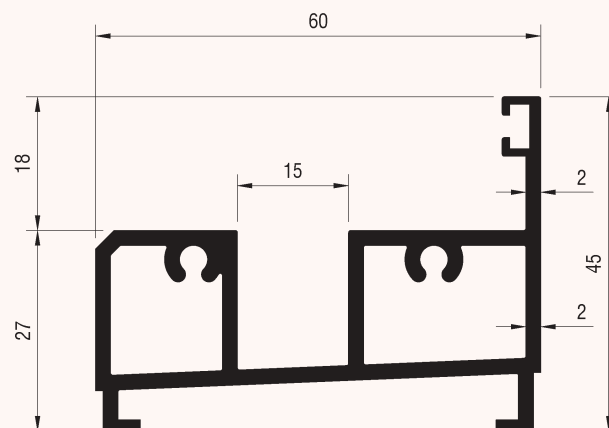
Profile Code : FD-6002 Unit Weight : 1.240 kg/m Perimeter : 289.2 mm
